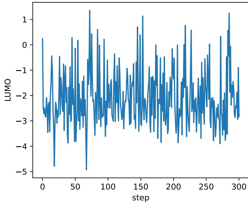
LUMO - evolution
