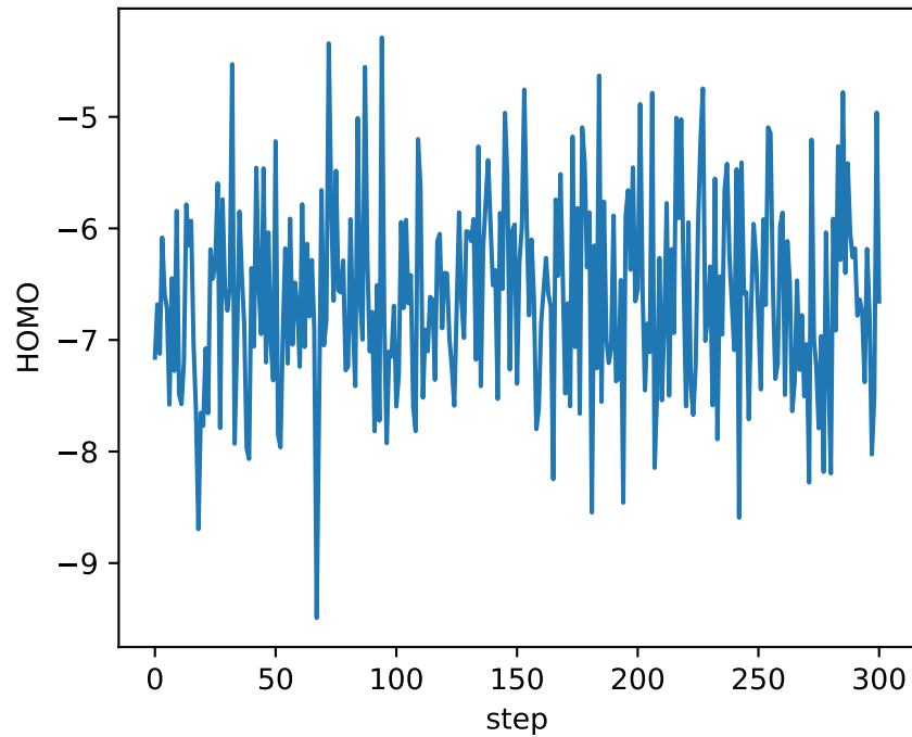
HOMO - evolution
